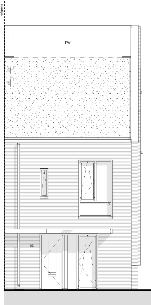
voorgevel
