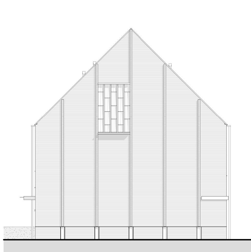
kopgevel met vleermuiskasten
