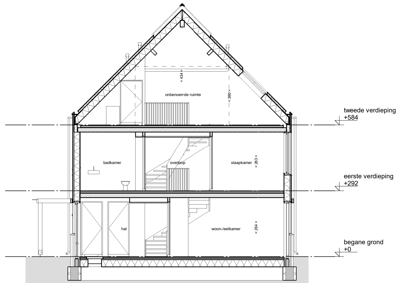
doorsnede
